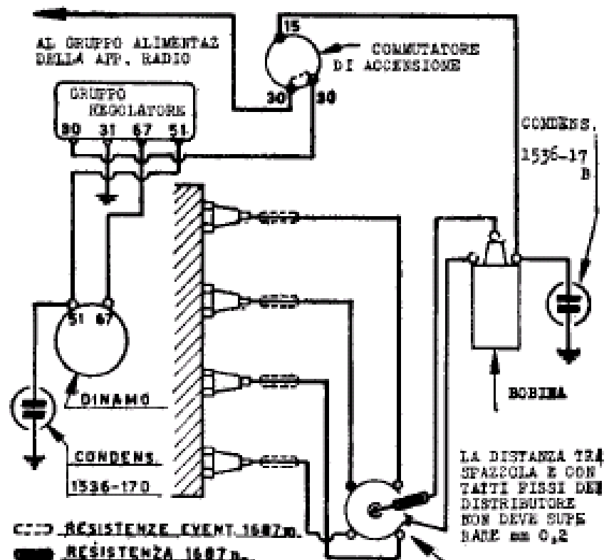
Fig. 26.23. - Autoradio CONDOR Mod. ULTRA PLAT. Soppressione dei disturbi su Fiat 1400.
